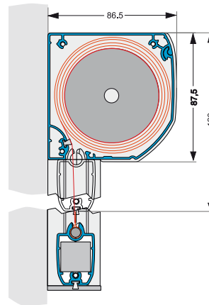
Befestigung der Seitenschienen
