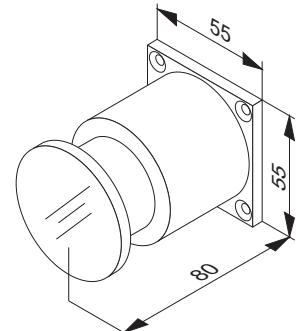
Teleskopanker mit Gegenplatte für GT 50 R xxx telescopic anchor with counterplate for GT 50 R xxx
