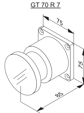
GT 70 R 7 Teleskopanker mit Gegenplatte für GT 70 R 2 telescopic anchor with counterplate for GT 70 R 2
