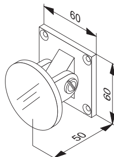
gefederte Gegenplatte für GT 50 R xxx, Schwenkbereich \pm 60^\circ spring loaded counterplate for GT 50 R xxx, swivelling range \pm 60^\circ
