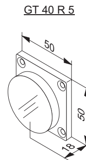
gefederte Gegenplatte für GT 40 R 18 spring loaded counterplate for GT 40 R 18
