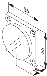
gefederte Gegenplatte für GT 50 R xxx spring loaded counterplate for GT 50 R xxx
