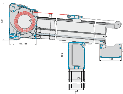
Ü1 Sparrenüberstand, außen Ü1s wie Ü1, mit Stahlverstärkung
