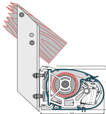
Dachsparren
