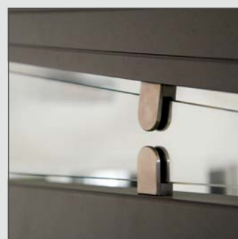
Option Dreiecksschluss mit Haltelaschen – optisch attraktive, „schwebende“ Befestigung
