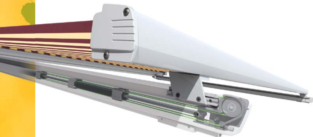
Ausfallprofil mit Nadellager gelagertem Fahrwagen.
