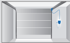
Antrieb in der rechten Torlaufschiene. Steuerung direkt neben dem Tor im Bereich des Seitenschlags.
